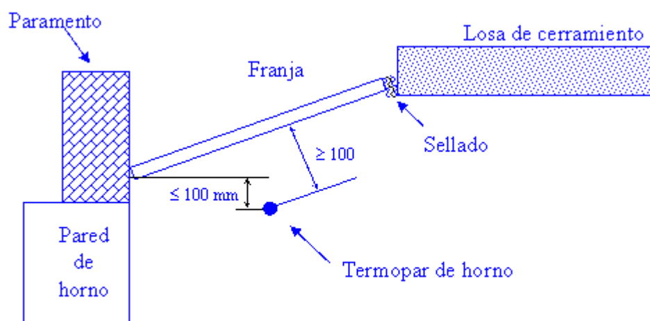
Figura 1.- Disposición Termopares de horno
